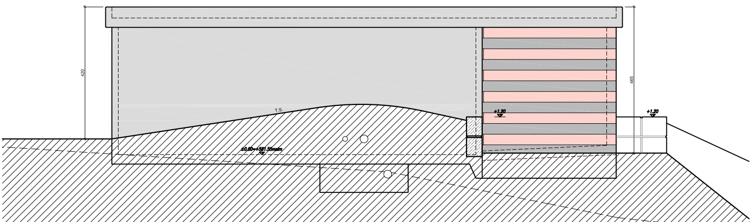
VISTA 2
