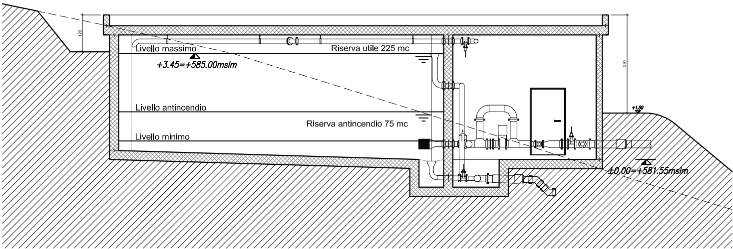
SEZIONE B-B
