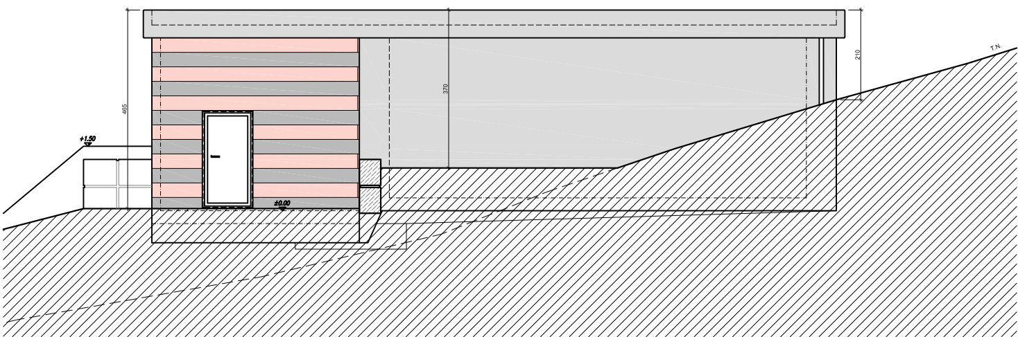
VISTA 1
