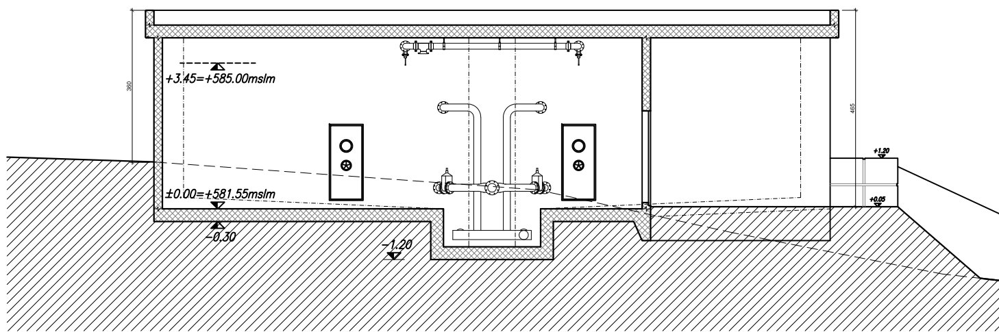
SEZIONE A-A
